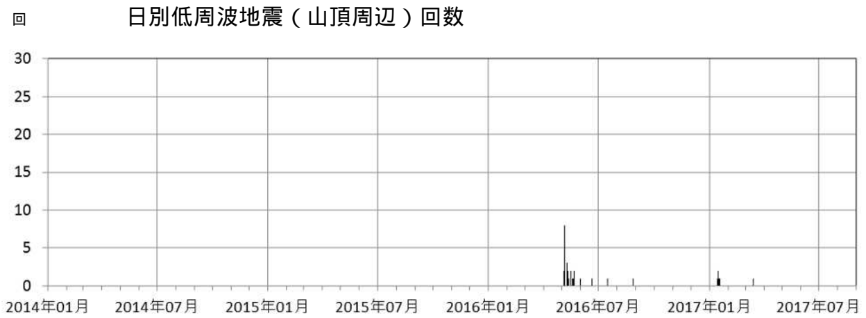
図 6 新潟焼山 日別地震回数（2014 年 1 月 1 日～2017 年 8 月 31 日）
