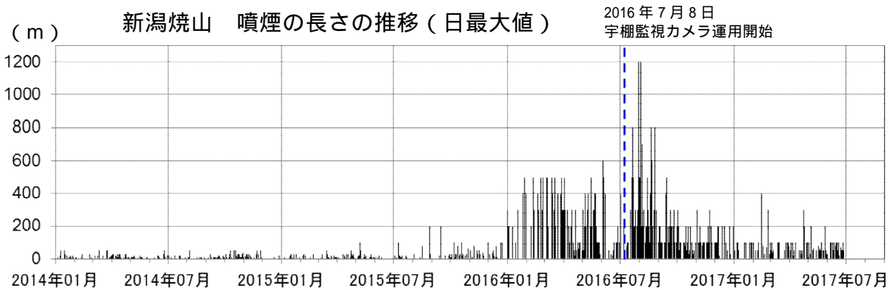
図4 新潟焼山 噴煙高度と噴煙の長さの推移 (それぞれ日最高値及び日最大値、2014年1月1日～2017年8月31日)
